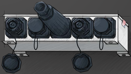
冷藏箱插座 如VARITAIN® PushIn Advance
